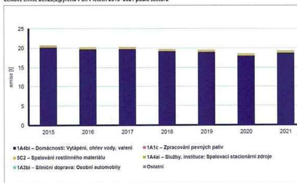
Celkové emise benzo[a]pyrenu v ČR v letech 2015–2021 podle sektorů
