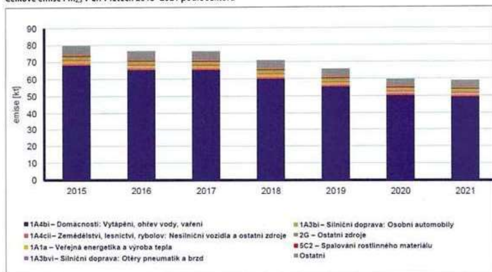
Celkové emise PM 2.5 v ČR v letech 2015–2021 podle sektorů
